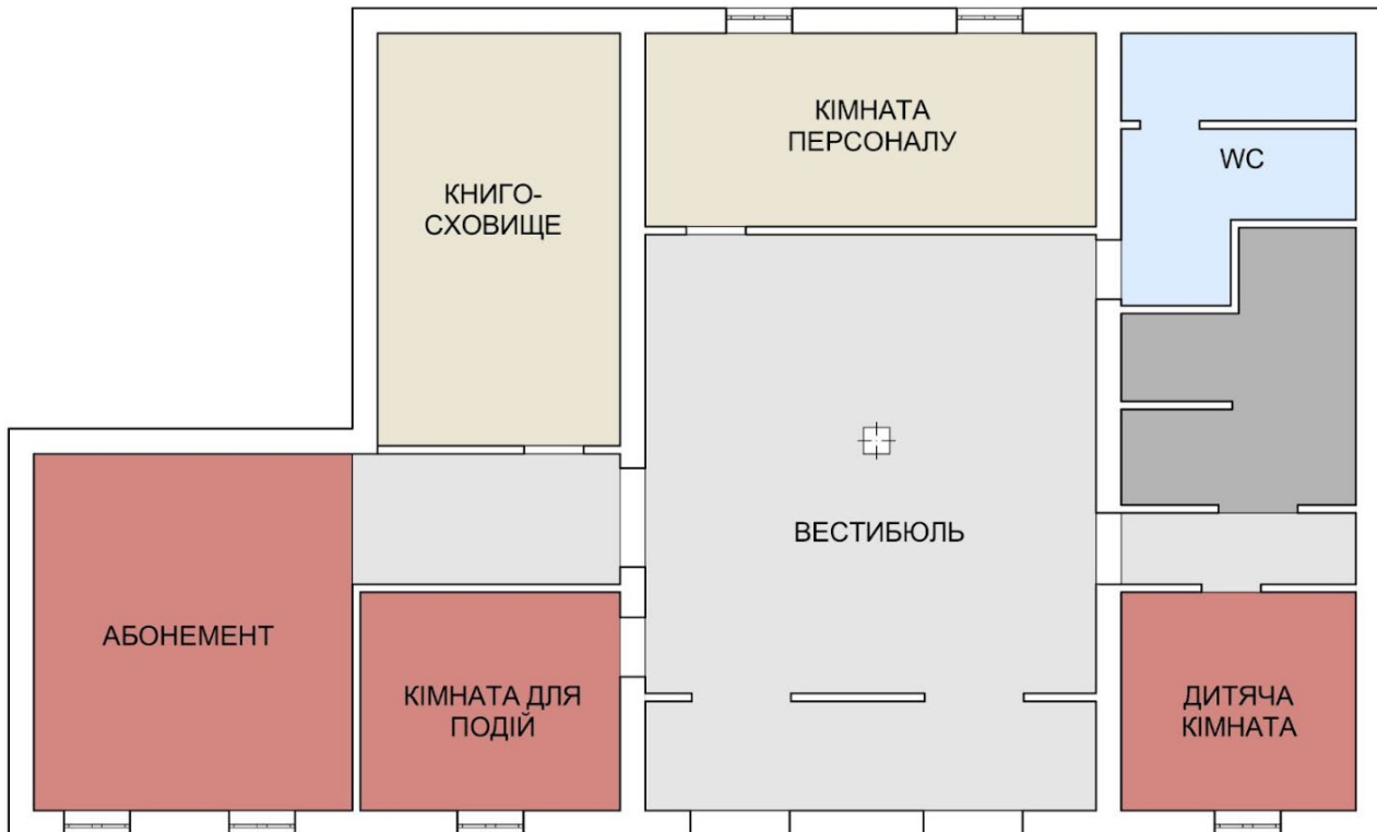
Існуючий план бібліотечного пункту.
